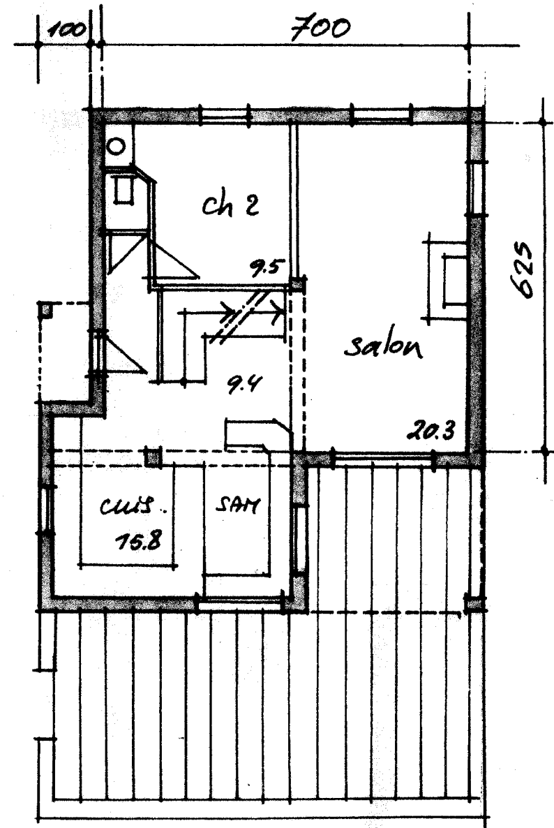
REZ-DE-CHAUSSEE
