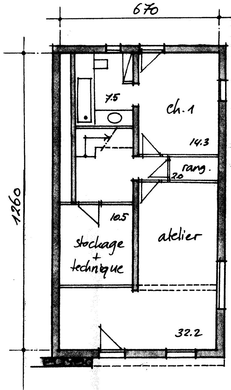
REZ-DE-JARDIN
